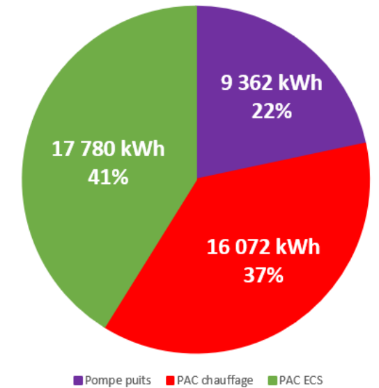
Répartition de la consommation électrique finale de la pompe de puits, de la PAC chauffage et de la PAC ECS
